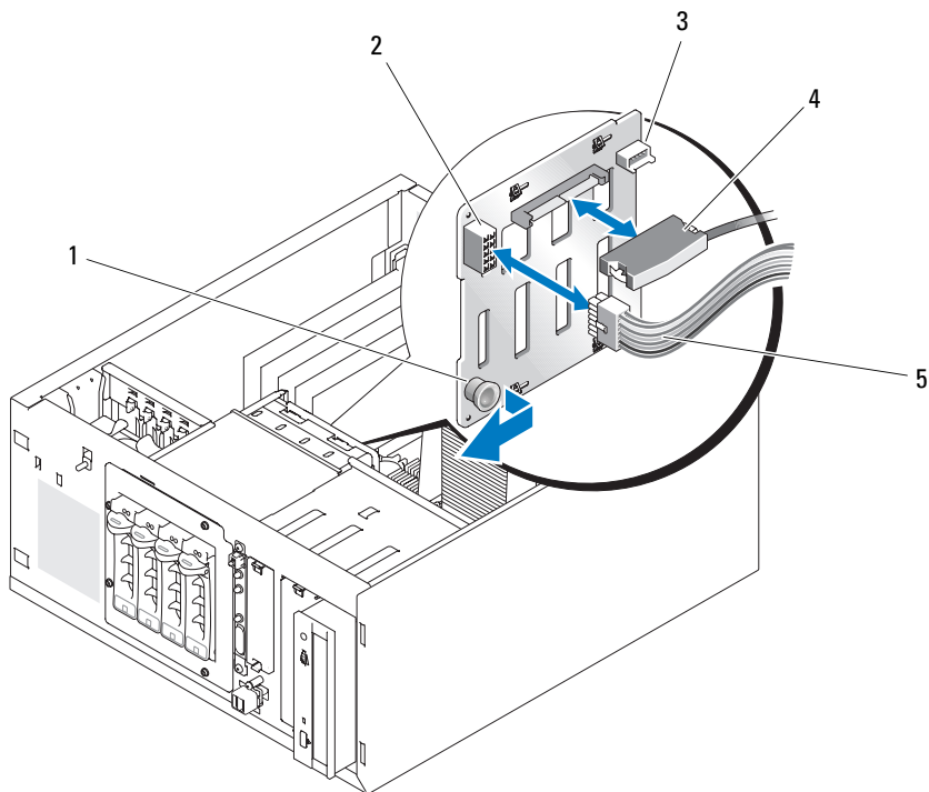
图 3-12. 安装 SAS 背板
