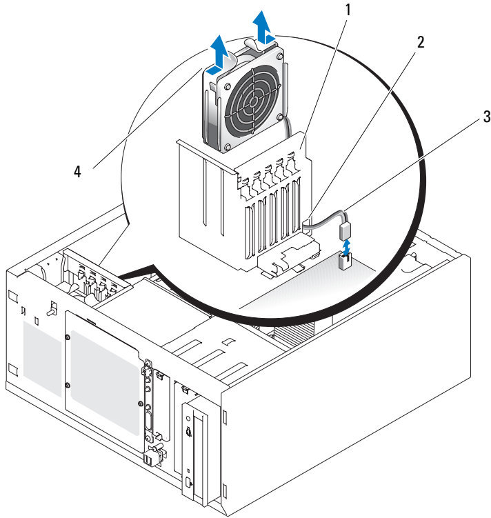
图 3-15. 前部系统风扇电源电缆
