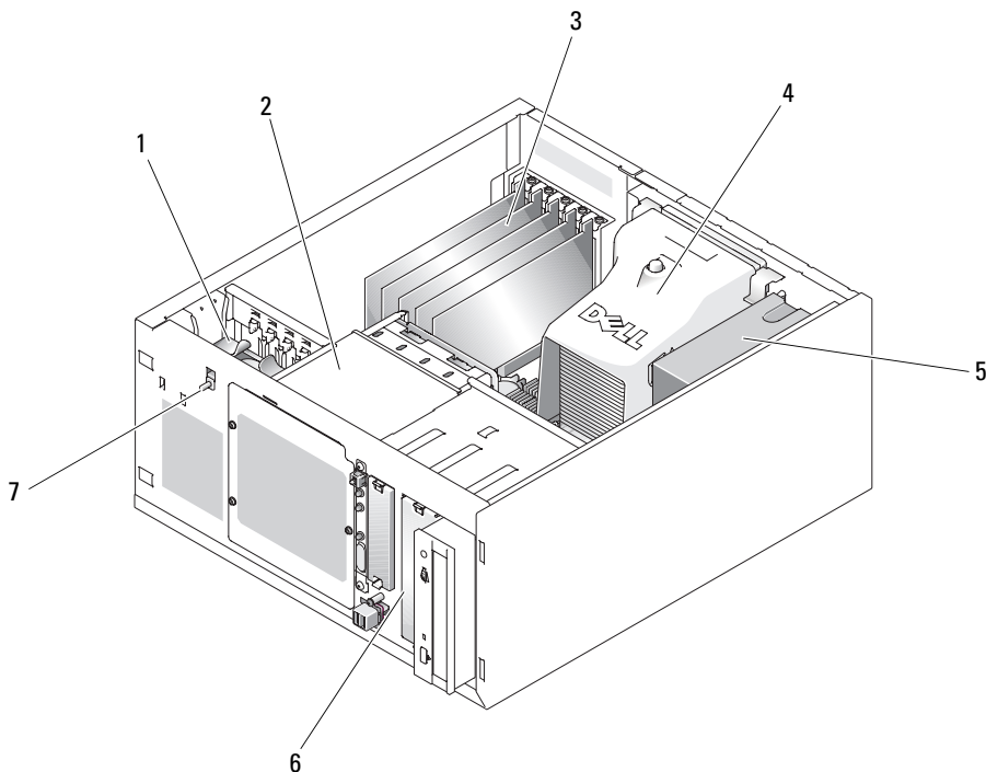
图 3-1. 系统内部组件
