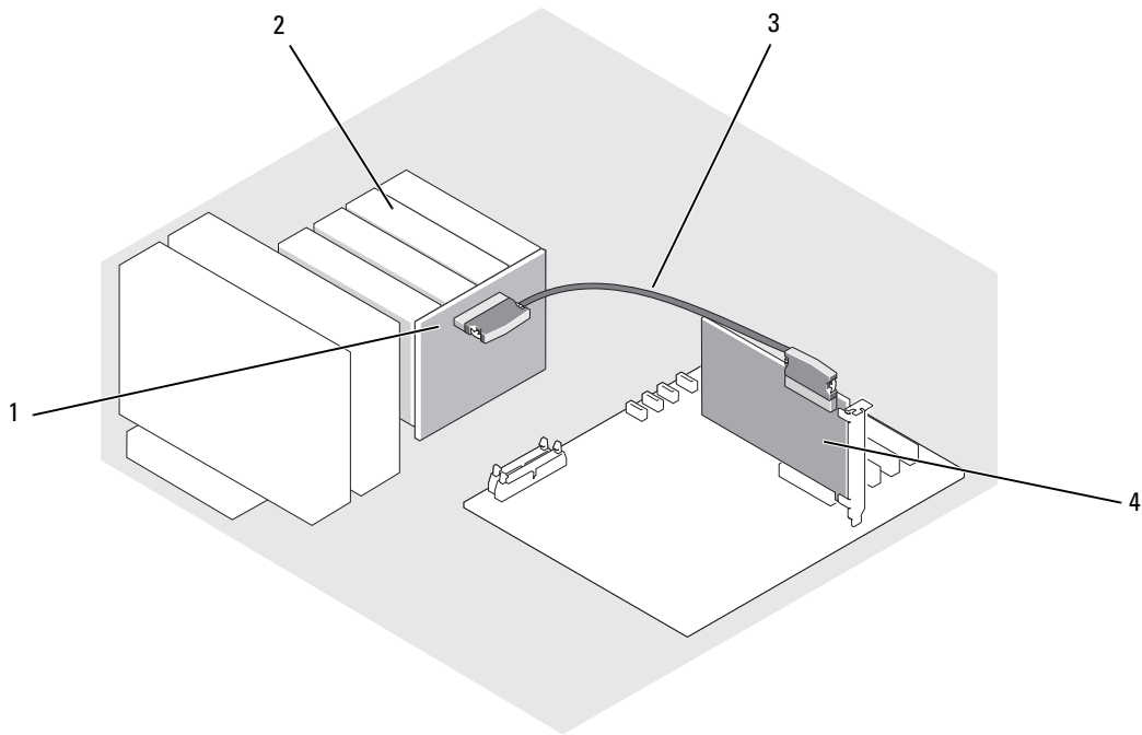
图 3-13. 连接至 SAS 控制器卡的 SAS 背板
