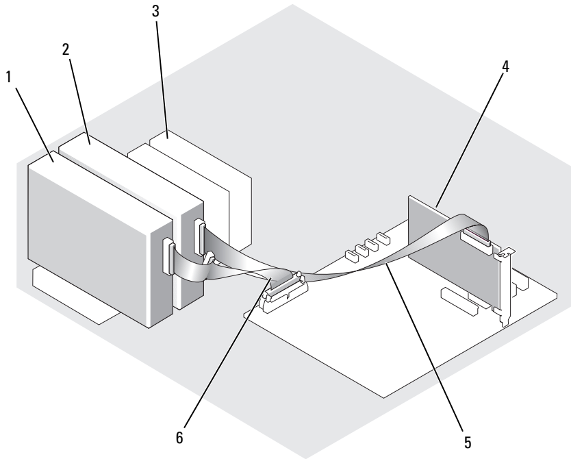
图 3-7. 将磁带驱动器连接至 SCSI 控制器卡
