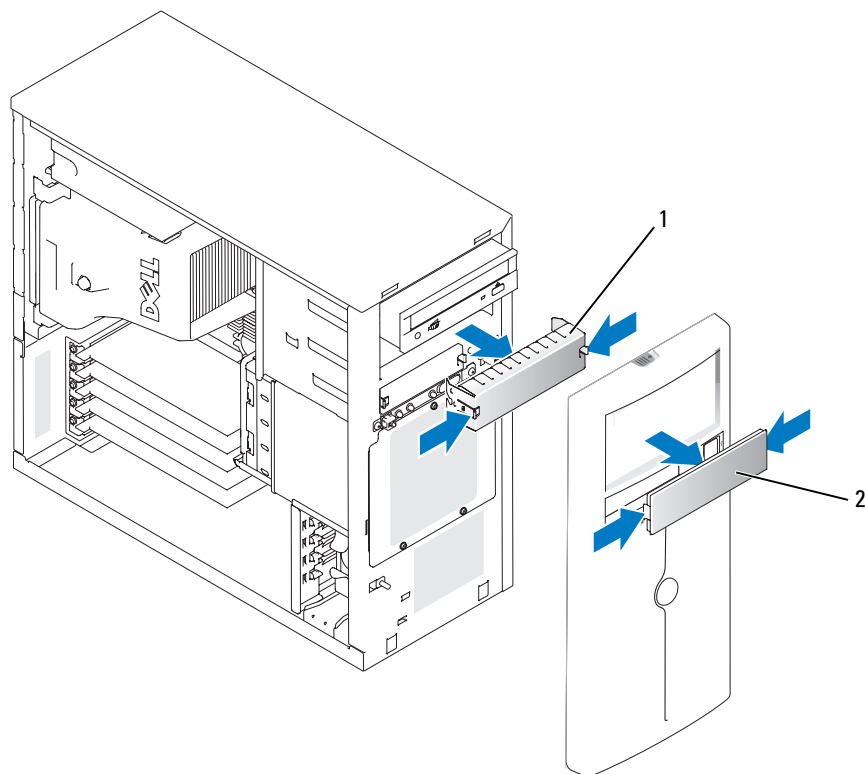
图 3-4. 卸下前面板驱动器插件
