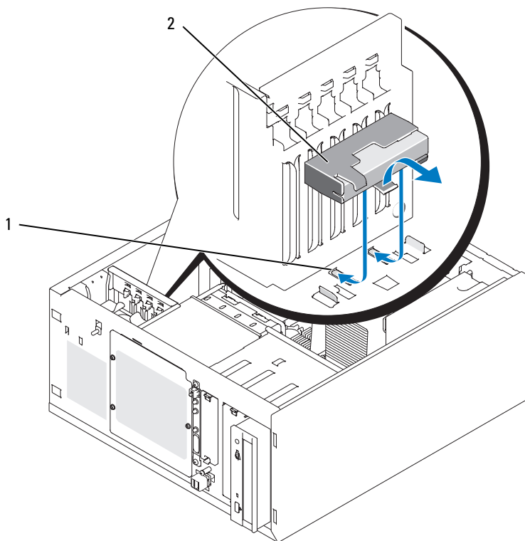
图 3-20. 更换 SAS 控制器卡电池
