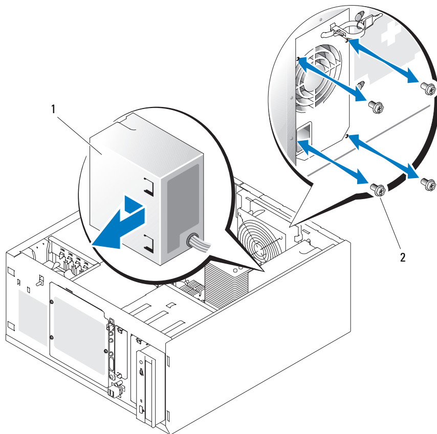
图 3-17. 卸下电源设备
