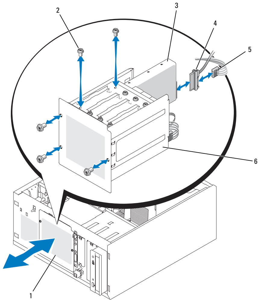
图 3-8. 安装或卸下硬盘驱动器
