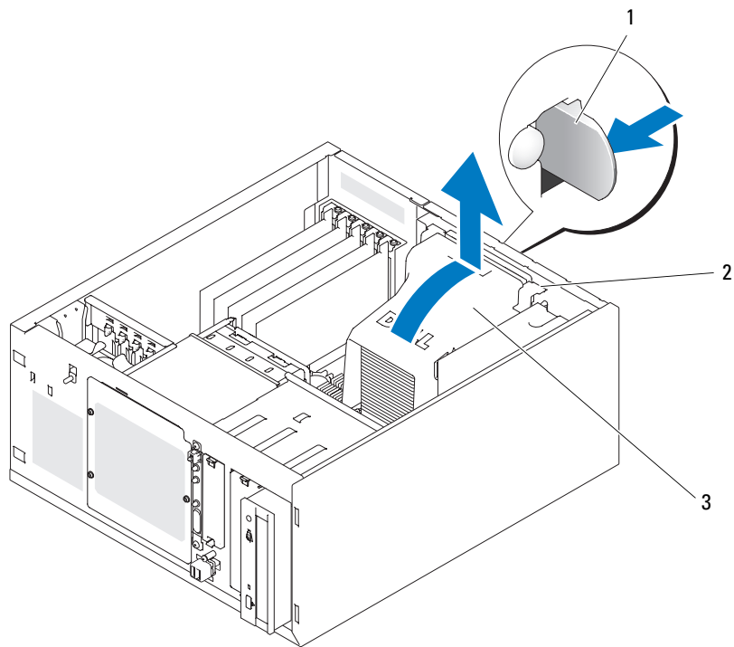
图 3-14. 卸下冷却导流罩
