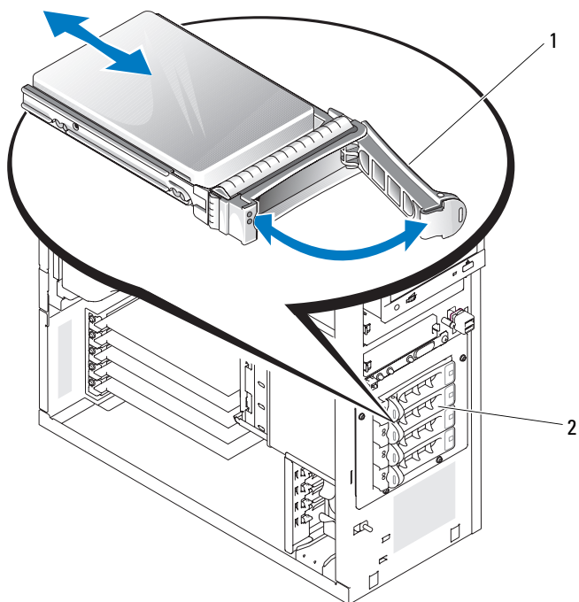
图 3-11. 卸下或安装 SCSI 硬盘驱动器托盘
