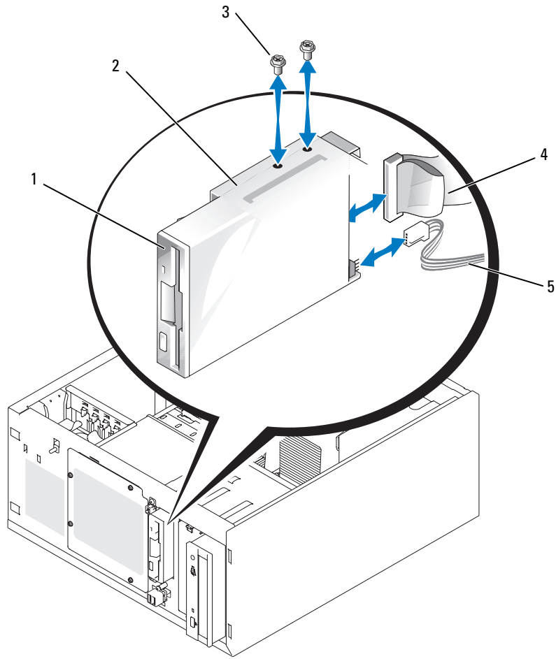
图 3-5. 卸下或安装软盘驱动器
