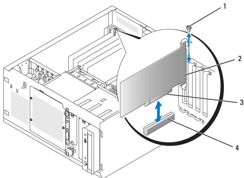
图 3-19. 卸下和安装扩充卡
