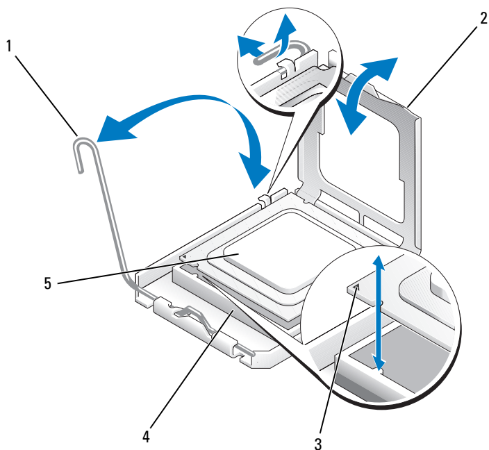
图 3-23. 卸下/更换处理器
