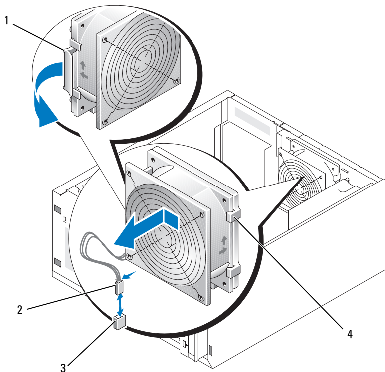
图 3-16. 卸下后部系统风扇
