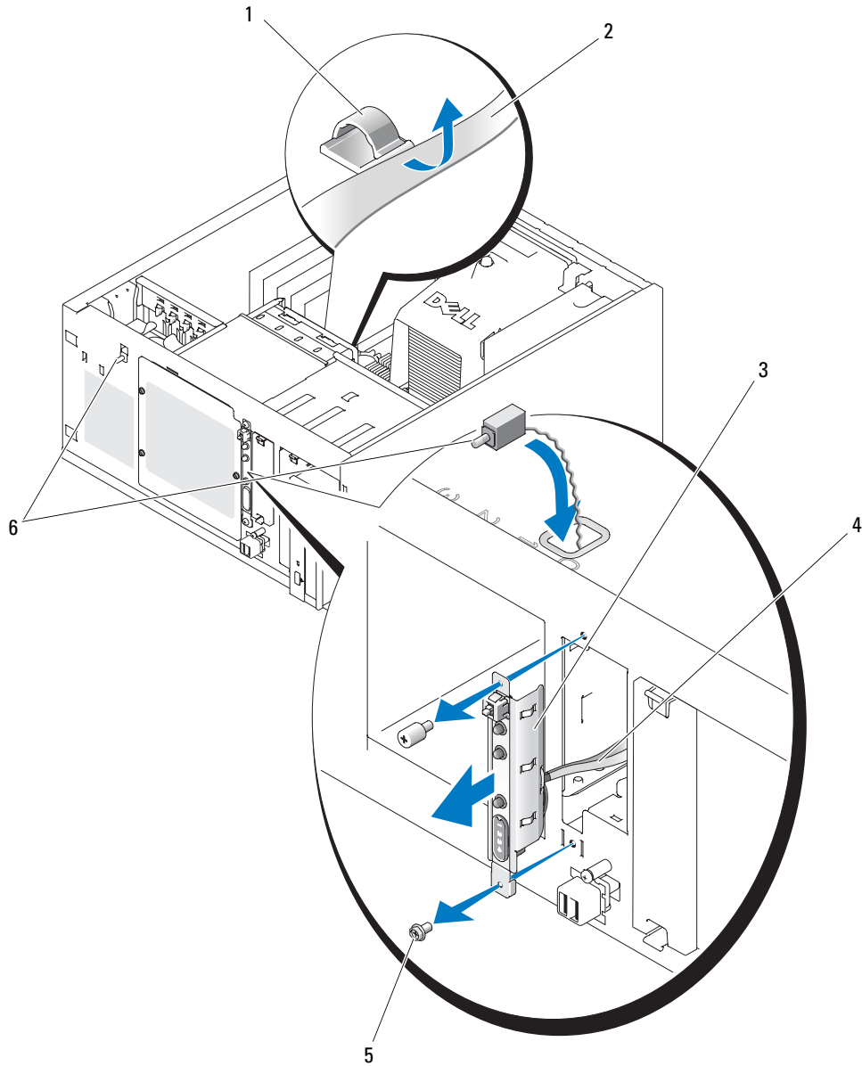
图 3-25. 卸下控制面板部件
