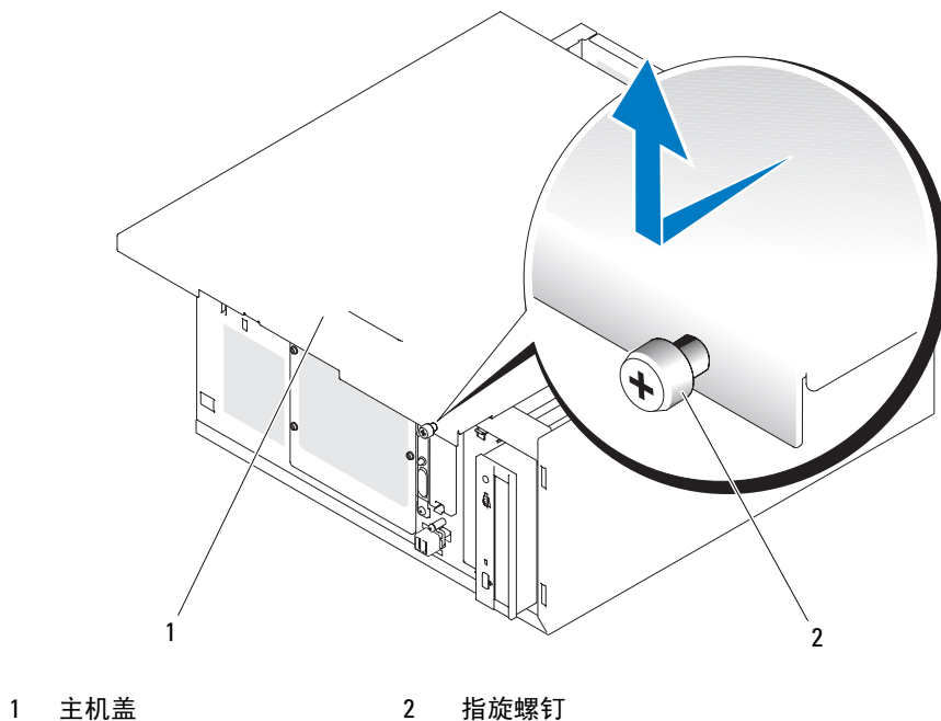
图 3-3. 卸下主机盖
