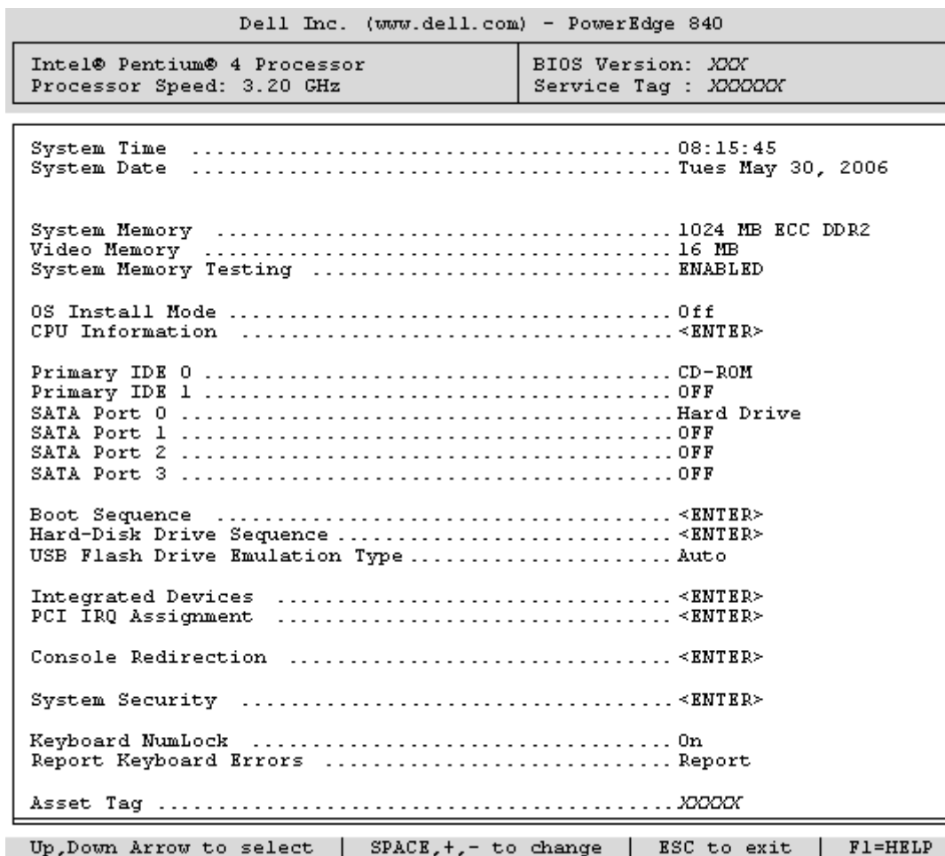
图 2-1. 系统设置程序主屏幕
